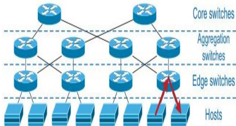
Рис. 1. Топология Fat Tree
