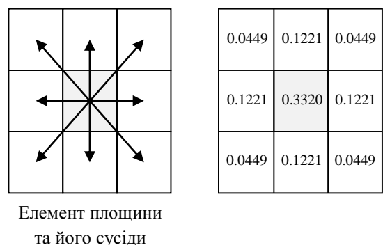
Рис. 2. Матриця розсіювання 3×3
