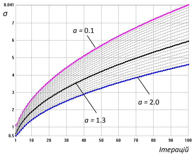
Рис. 3. Залежність \sigma від кількості ітерацій для матриці 3 \times 3
