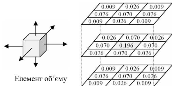
Рис. 1. Куб розсіювання 3×3×3
