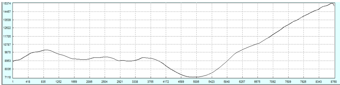
Рис. 6. Графік тренду, виділеного методом “Гусениця-SSA”
