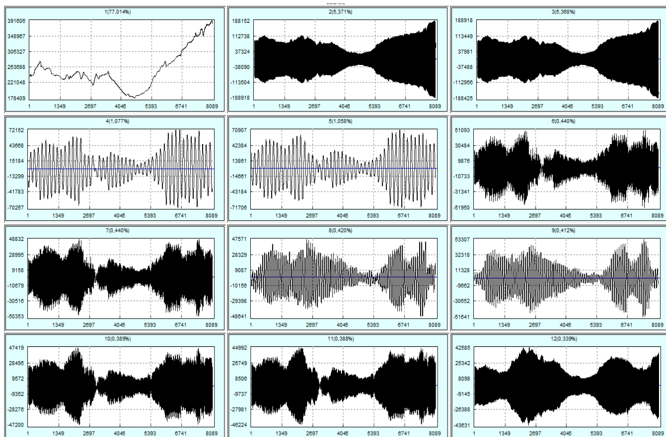
Рис. 2. Графіки перших 12 компонент, отриманих після розкладу часового ряду методом "Гусениця-SSA"
