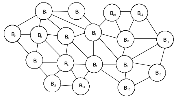
Рис.1. Структура графа
